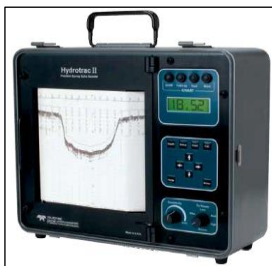
Figura 6. Ecosonda Hidrotrac II
